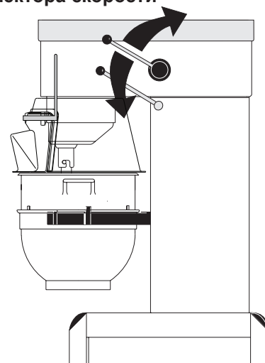
Рис. 4 Рычаг селектора скорости
