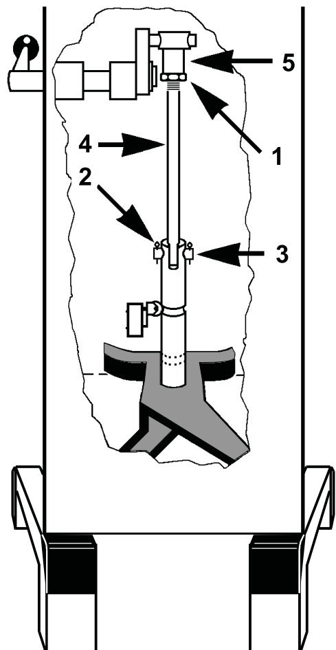
Рис. 7b Регулировка высоты дежи:
