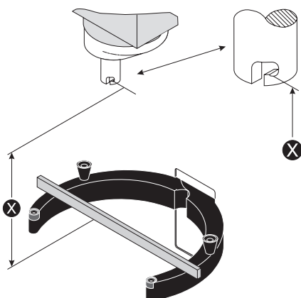
Рис. 7а Измерение высоты дежи X:
